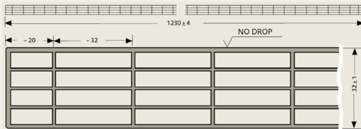
Querschnitt der PLEXIGLAS® Heatstop Cool Blue S5P 32 (Maße in mm)
